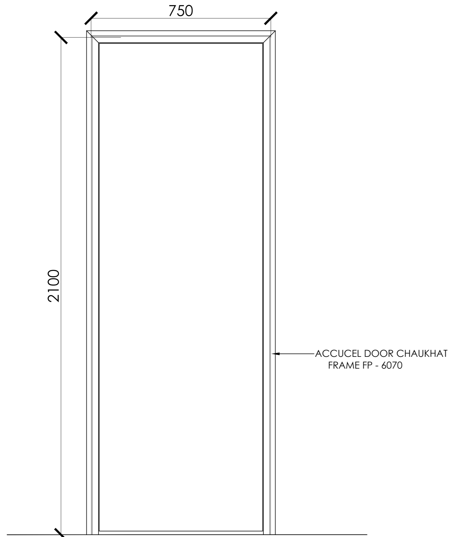
FRAME ELEVATION
